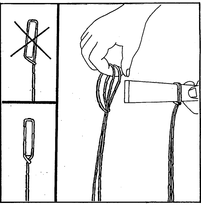
Maak lussen voor de aanbindlatten Make loops for the apron and warp bar Mache eine Schlaufe für die Anbindelatten
