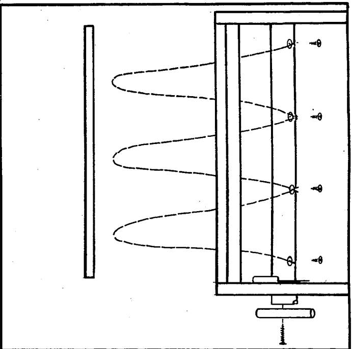
Koorden voor de aanbindlatten Cords for the apron and warp bars Kordel für die Anbindelatten
